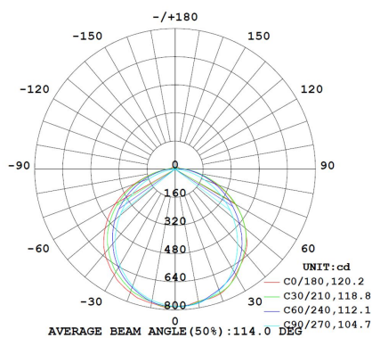
Photométrie ABE06T20WC850
