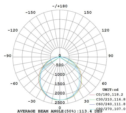
Photométrie ABE15T54WC850
