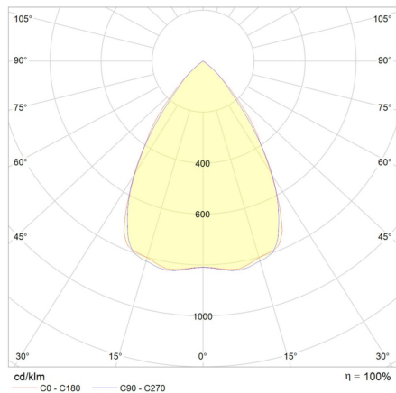
Photométrie AHD100W 4000°K
