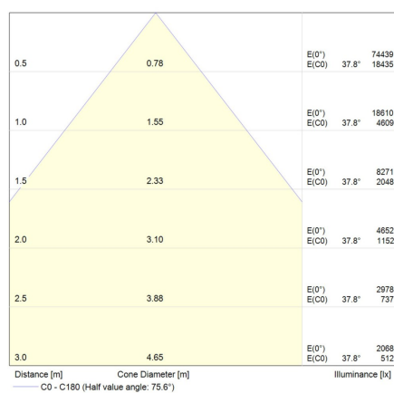
Cône de performance AHD200W 4000°K
