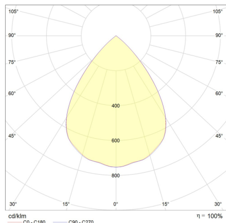
Photométrie AHD200W 4000°K
